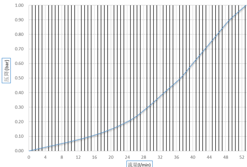
MTC08 流量曲线
